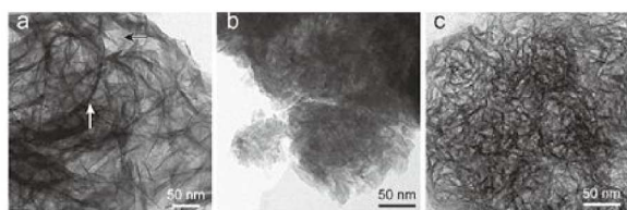
図1：透過電子顕微鏡画像。(a)細胞産生骨アパタイト(白：ナノファイバー、黒：薄板)。(b)従来法で作製した ACP から相転移したアパタイト。(c)独自の方法で作製した新構造 ACP から相転移したアパタイト。
